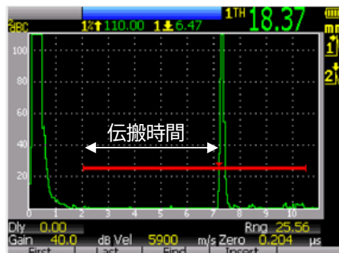
図-1 測定結果
